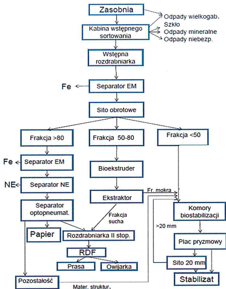
Rysunek 2. Schemat technologiczny Zakładu Unieszkodliwiania Odpadów w Lubawce.
