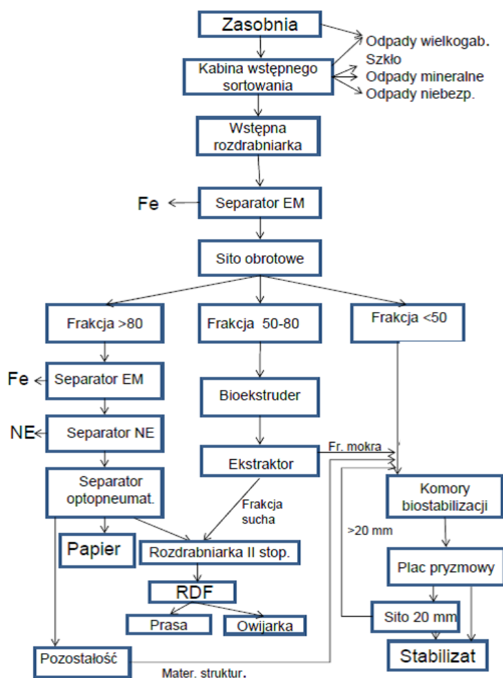
Rysunek 2. Schemat technologiczny Zakładu Unieszkodliwiania Odpadów w Lubawce.
